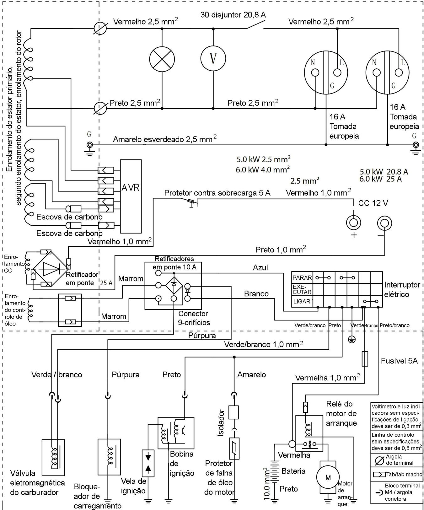
Diagrama Elétrico Esquemático FG7000RE
